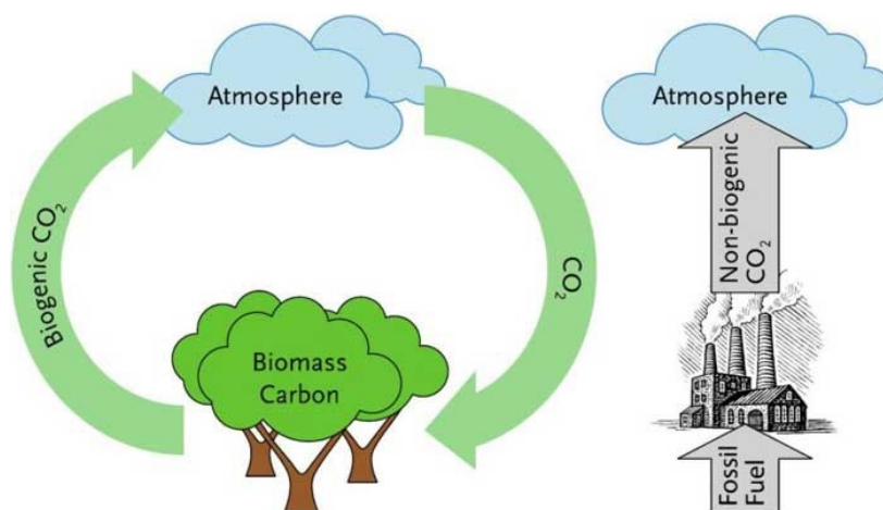
Figura 1. Tipo de emisiones de CO 2 . Fuente: https://www.forestalmaderero.com/articulos/item/que-es-el-carbono-biogenico.html
